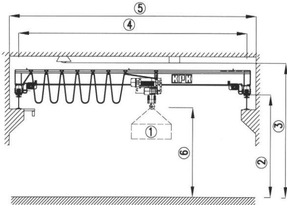
JEDNONOSNÍKOVÝ ŽERIAV
