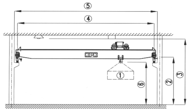
DVOJNOSNÍKOVÝ ŽERIAV
