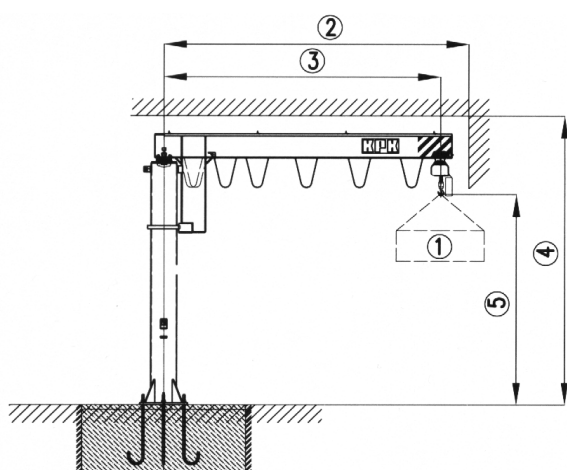
STĽPOVÝ ŽERIAV
