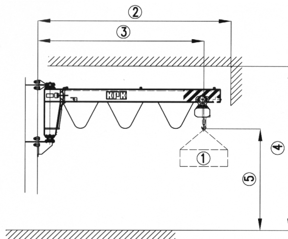
KONZOLOVÝ ŽERIAV
